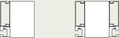
Pfosten + Führung + Ausgleichsprofil / Post + guide rail + compensation profile
