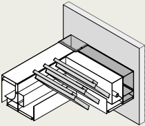
Wandmontage mit Profil / Wall mount with profile
