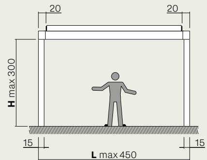
Vorderansicht / Front view
