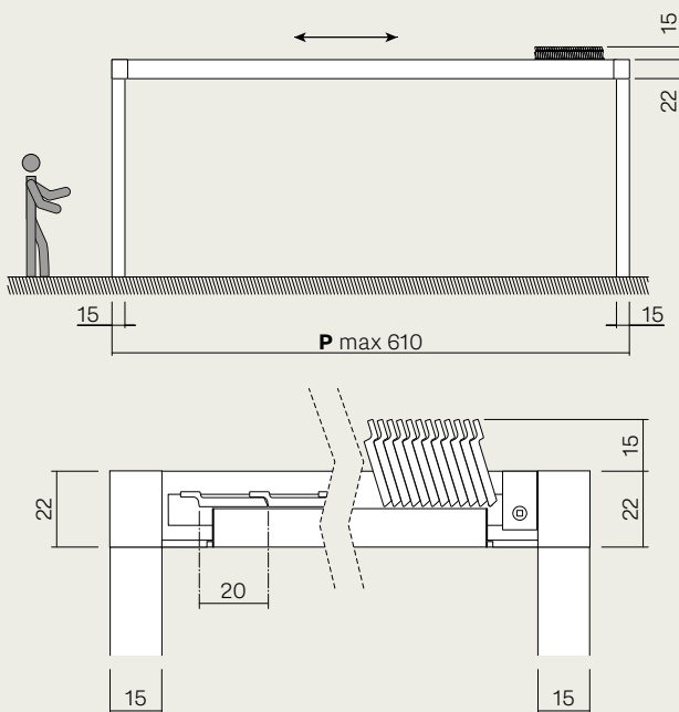
Seitenansicht / Side view
