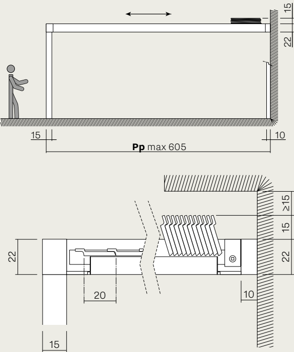
Seitenansicht / Side view
