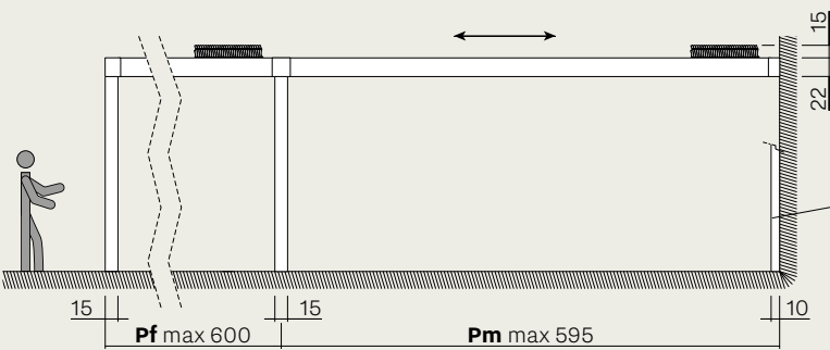
Seitenansicht / Side view
