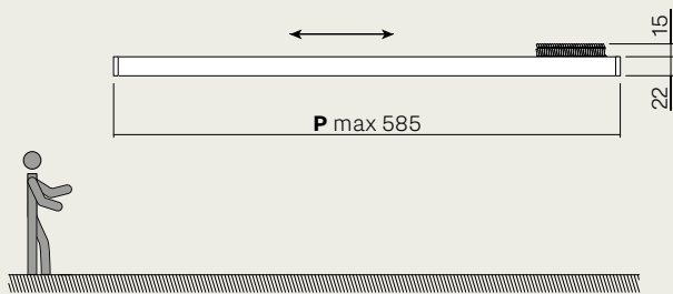
Seitenansicht / Side view
